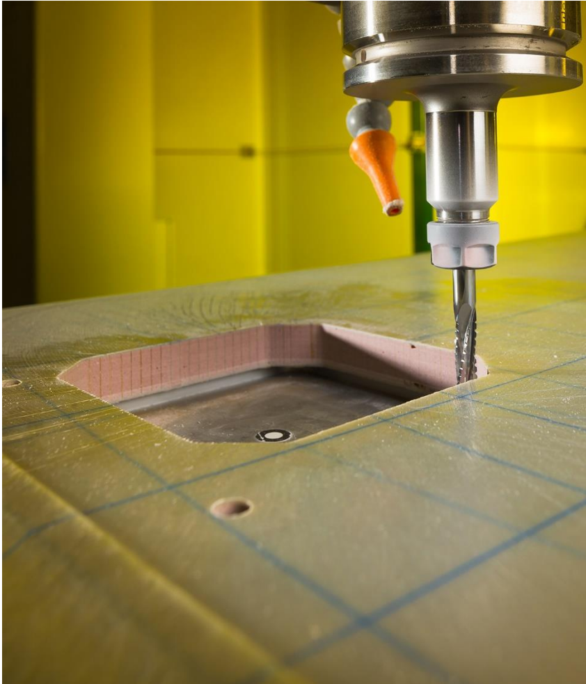
Bearbeitung mit 5-Achsen-CNC-Bearbeitungszentren
